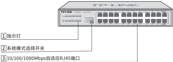
图1-1 前面板示意图
